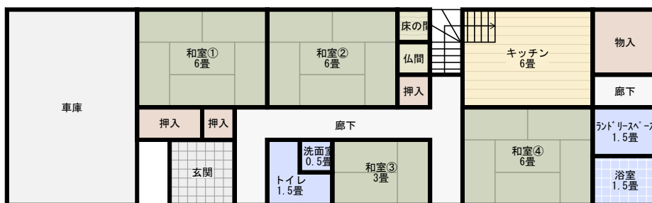
2 階 縮尺 1/150
