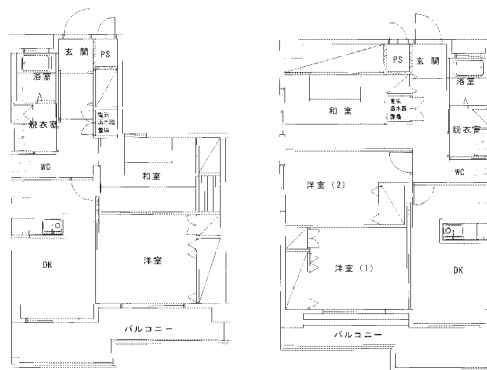
間取り図 2DK（左）と3DK（右）
