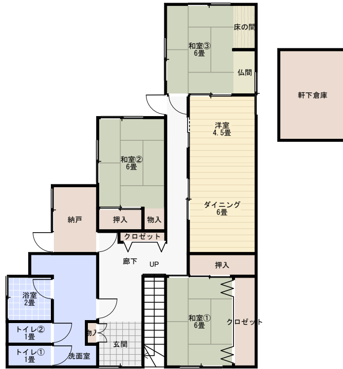
2階 縮尺 1/150
