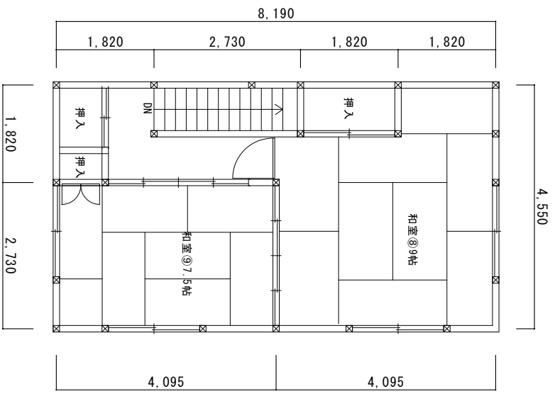
2階平面図
