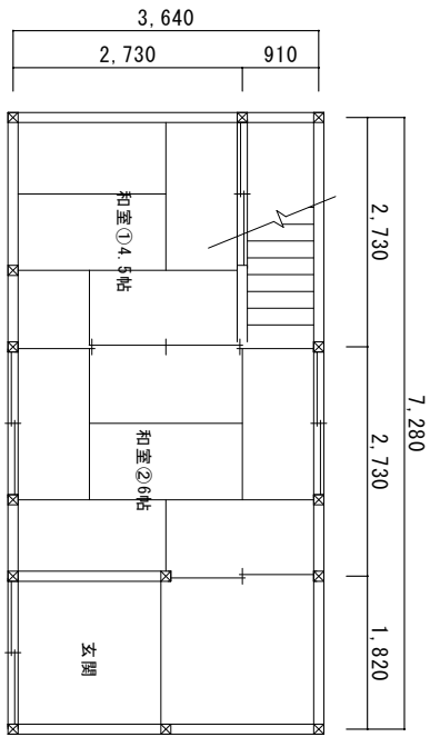
離丸 2階平面図
