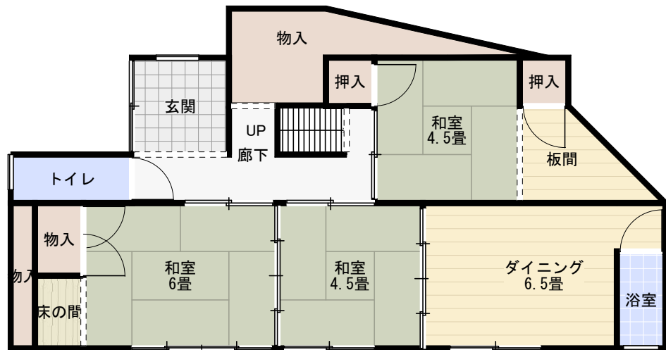
1階 縮尺 1/100
