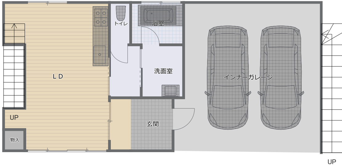
1階縮尺 1/100
