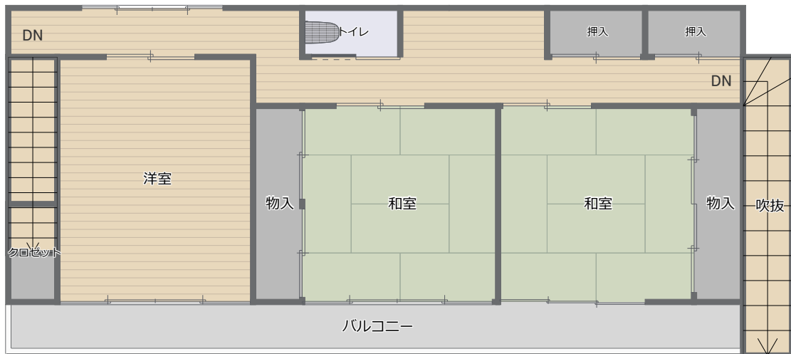
2階縮尺 1/100
