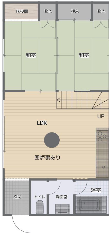
2階縮尺 1/100
