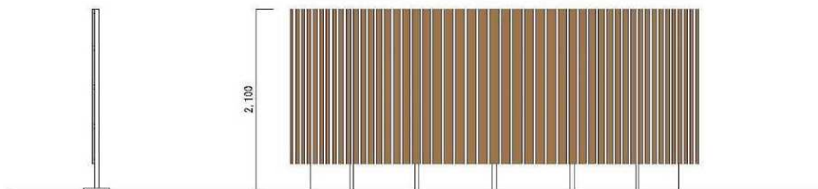
立面図
