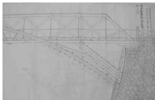
写真：明治時代の浅水橋設計図
