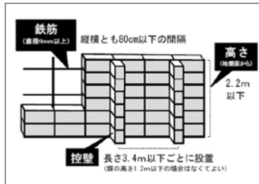
▲補強コンクリートブロック塀のイメージ図
