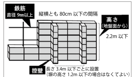
▲補強コンクリートブロック塀のイメージ図
