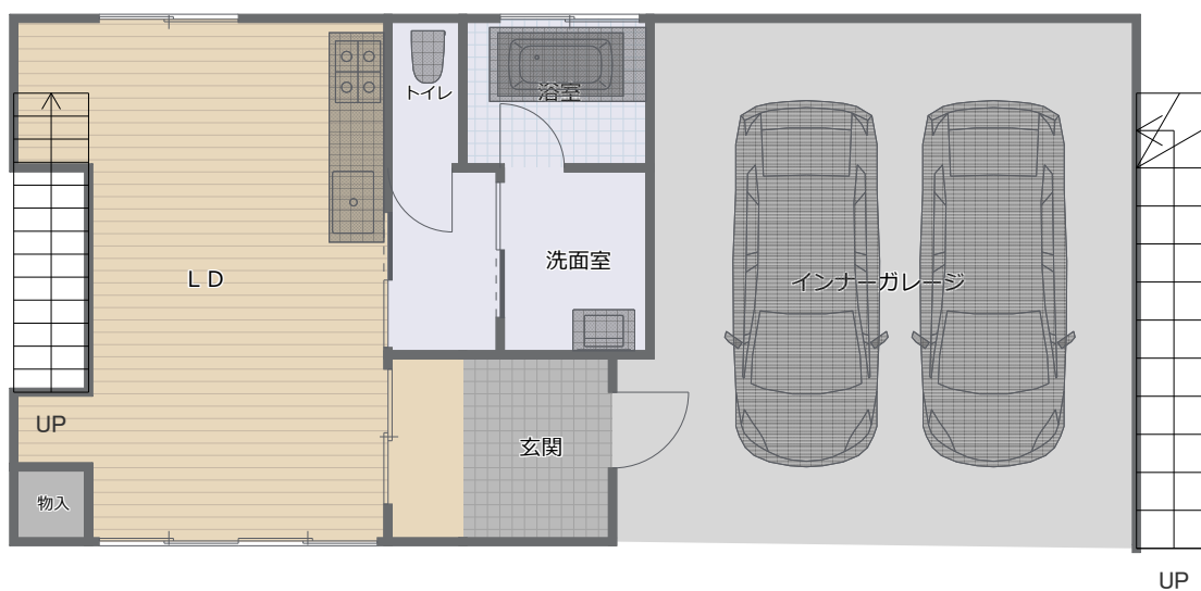
1階縮尺 1/100
