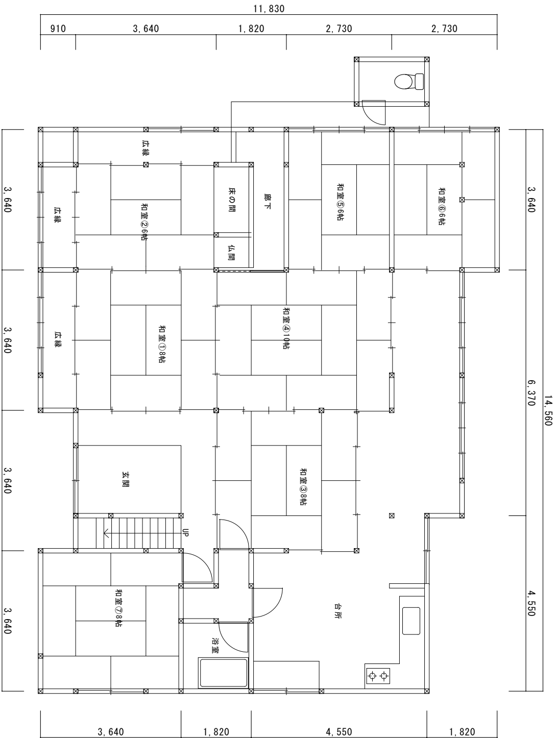
1階平面図
