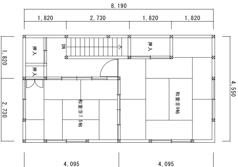
2階平面図
