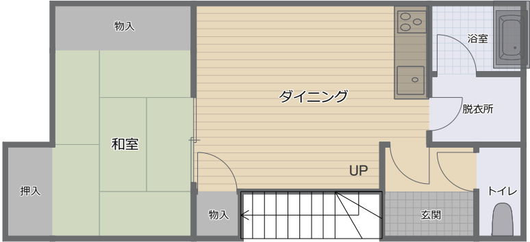
1階縮尺 1/100
