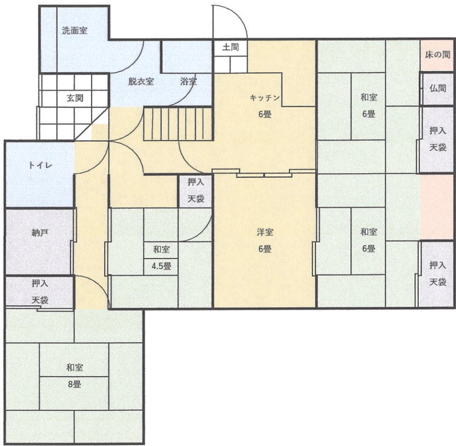
1階 縮尺1/100
