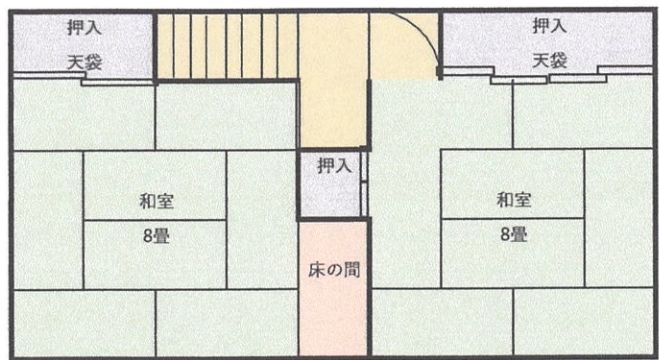
2階 縮尺1/100
