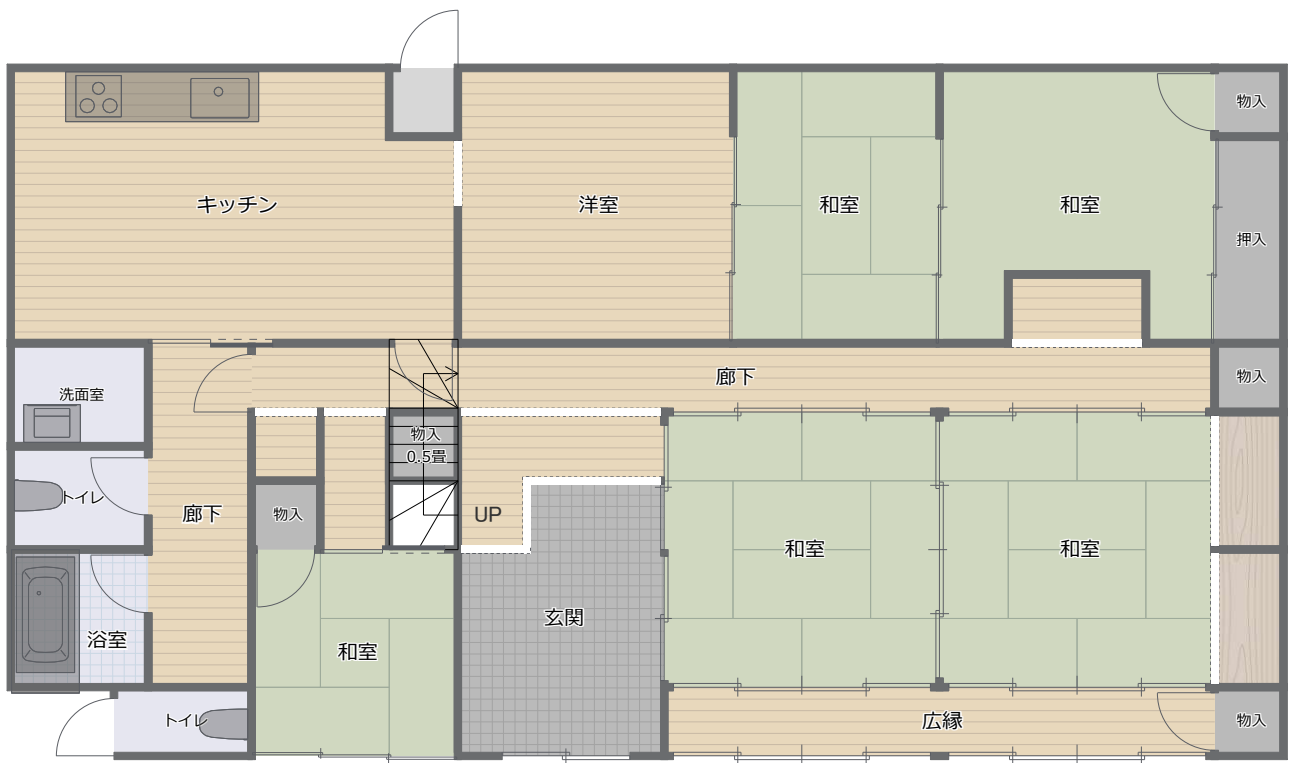
1階縮尺 1/100
