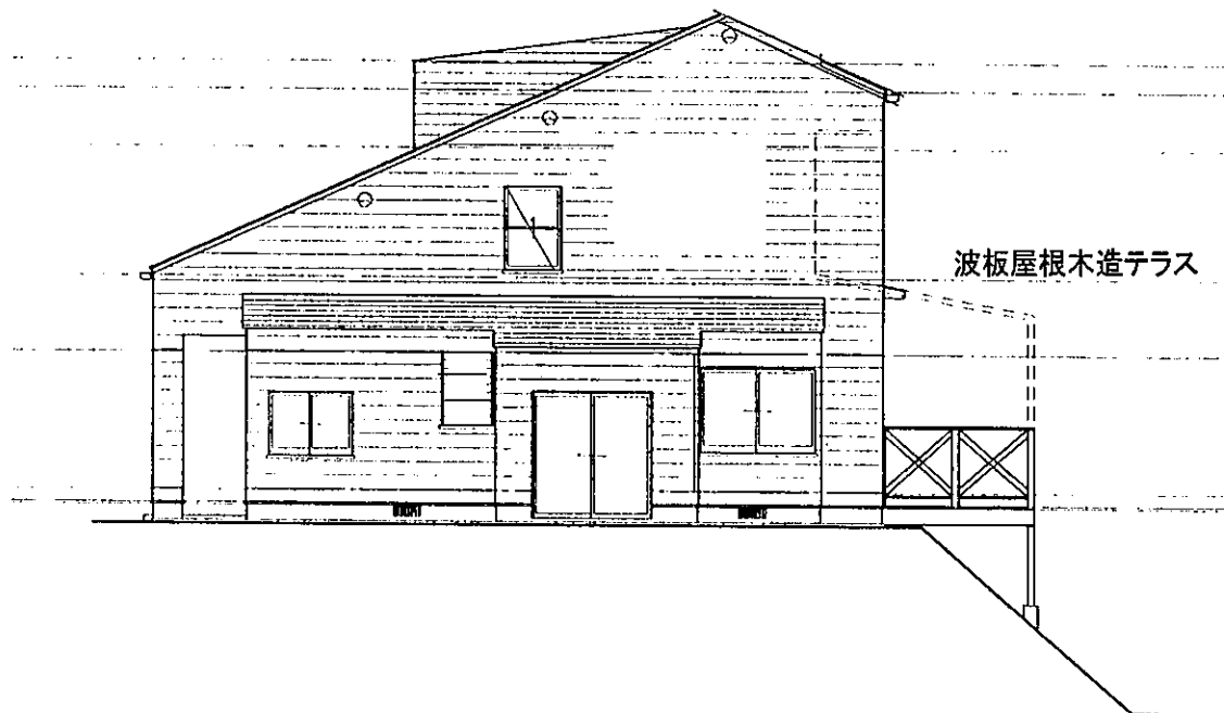
北 立 面 図
