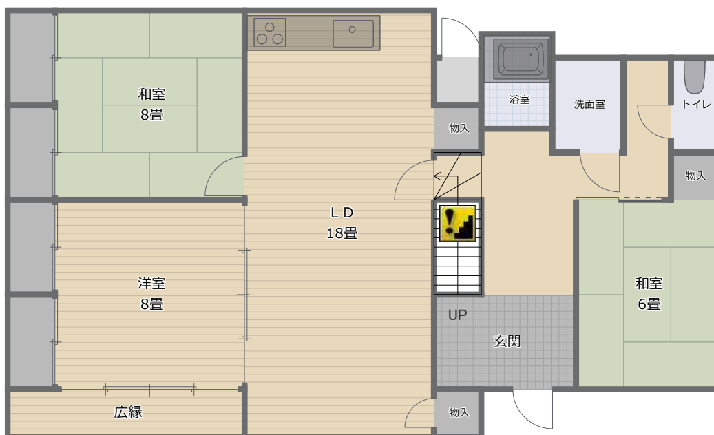
1階縮尺 1/100
